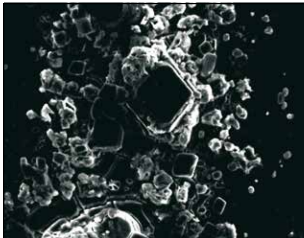
Kalkablagerungen mit Wellan behandeltes Wasser. Vergrößerung: 250-fach
